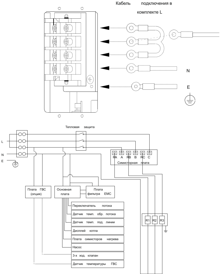
Рис. 10. Схема однофазного подключения
