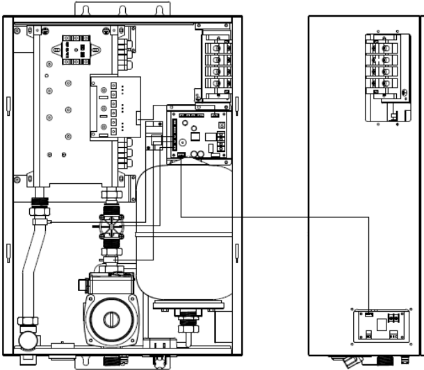
Рис. 13. Схема монтажа платы ГВС
